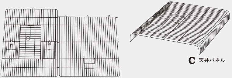
A 前面パネル+右側面パネル (接続済)
